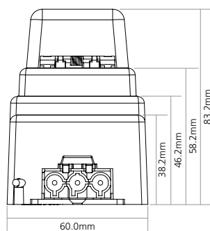
RCD Module
